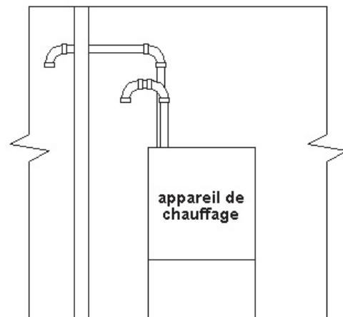
Figure 7 - Apport indirect d'air nécessaire à la combustion
