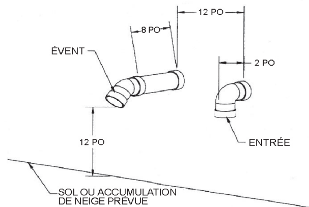
Figure 32 - Dégagement par rapport à la neige
