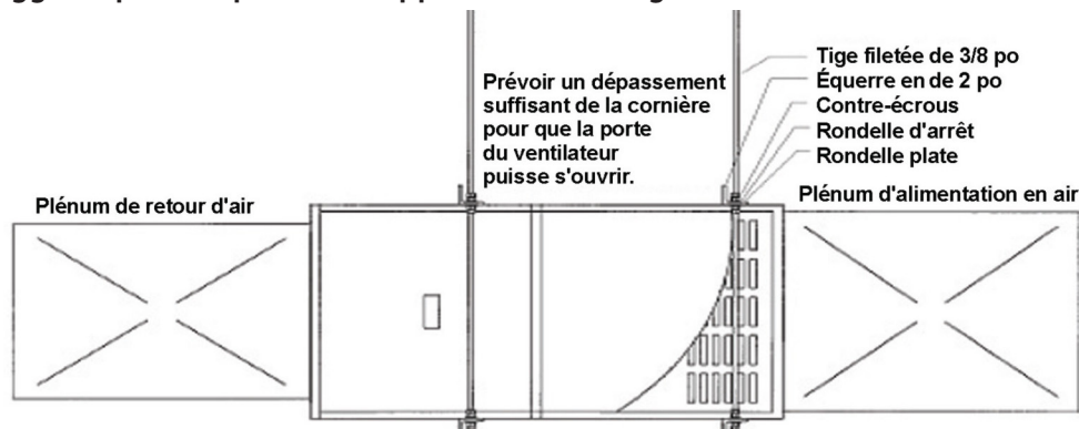
Figure 3 - Méthode suggérée pour suspendre un appareil de chauffage horizontal
