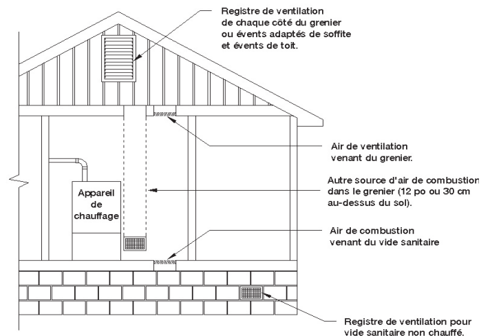
Figure 5 - Air extérieur pour combustion, grenier ou vide sanitaire (cas 3)
