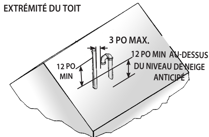
Figure 11 - Détail de l'installation de ventilation verticale type
