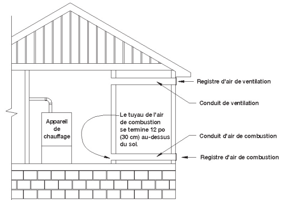
Figure 6 - Air extérieur pour combustion, horizontal (cas 4)
