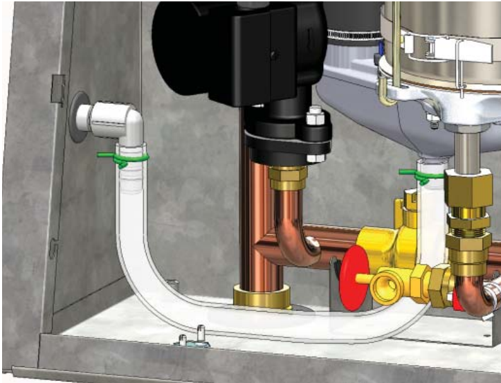
FIGURE 5-1 Tuyau d'écoulement de la condensation
