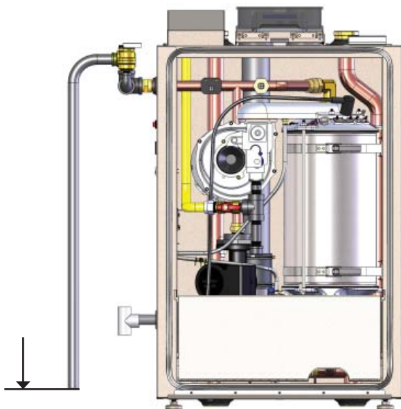
FIGURE 5-2 Canalisation de sortie de la soupape de sûreté
