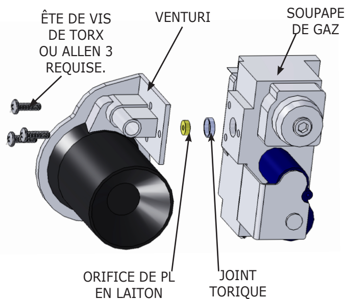
Figure 1 : Détacher le corps du module Venturi de la soupape de gaz
