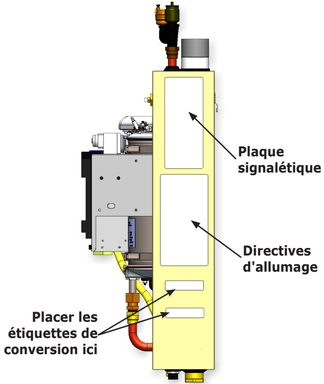
Figure - 4 Emplacement de l'étiquette de conversion 050/075/100/150/200
