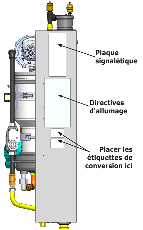
Figure - 5 Emplacement de l'étiquette de conversion, 299
