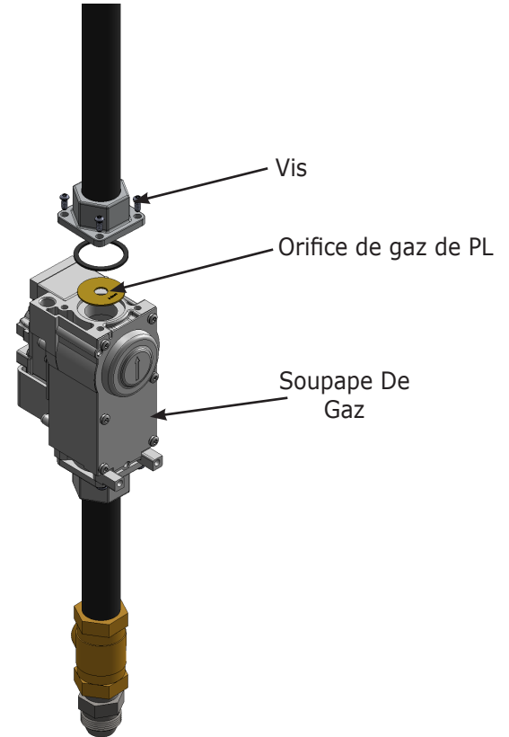
Figure - 2 Débrancher du Distributeur gaz bride supérieure - 299
