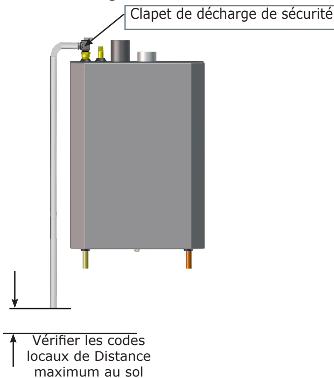
FIGURE 6-2 Clapet de décharge de sécurité tuyauterie de décharge
