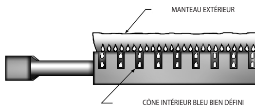
Figure 16 - Brûleur
