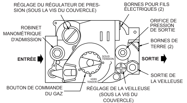
Figure 14- Soupape de gaz automatique
