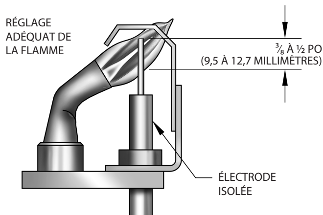
Figure 15 - Flamme de la veilleuse
