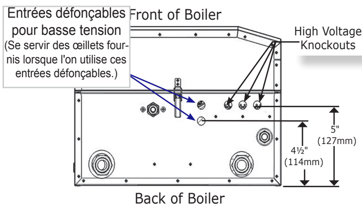
FIGURE 8-1 Entrées défonçables au bas de la chaudière
