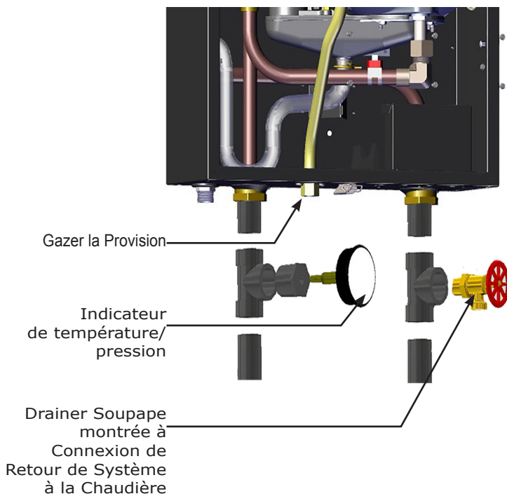
FIGURE 5-3 Installation de l'indicateur de température/pression
