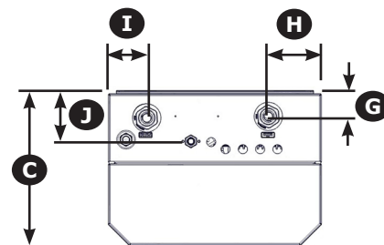
Vue de dessous dimensions 150-299 MBH
