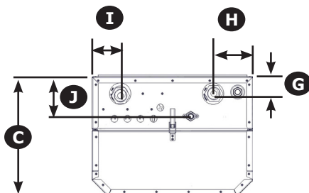
Vue de dessous dimensions 50-100 MBH
