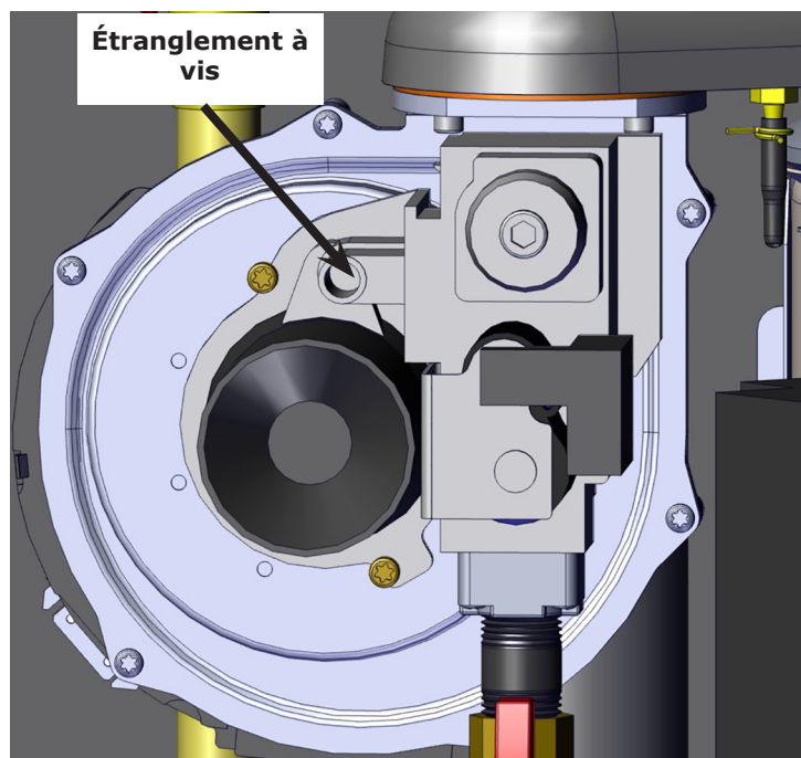
FIGURE 9-3 Soupape de gaz : modèle 050/075/100/150/200 MBH
