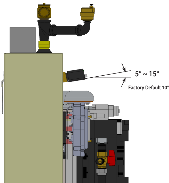
FIGURE 4-3 Faible Coupure Eau Orientation
