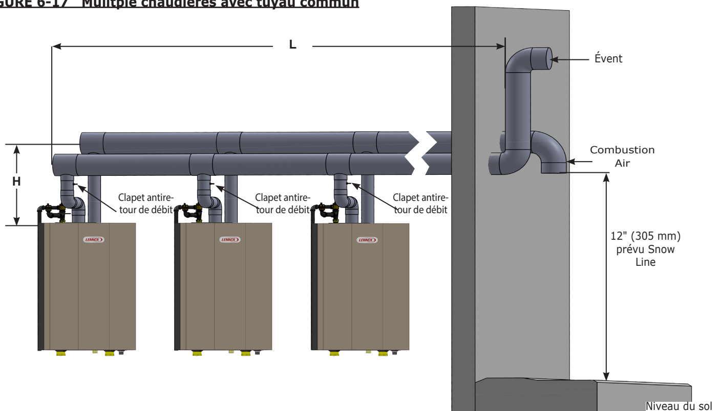
FIGURE 6-17 Multiple chaudières avec tuyau commun
