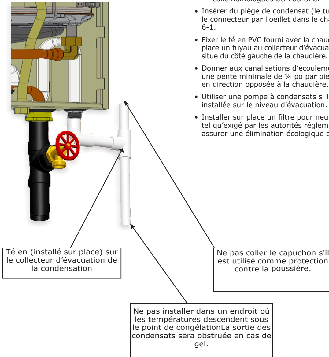
FIGURE 6-21 Tuyau d'écoulement de la condensation
