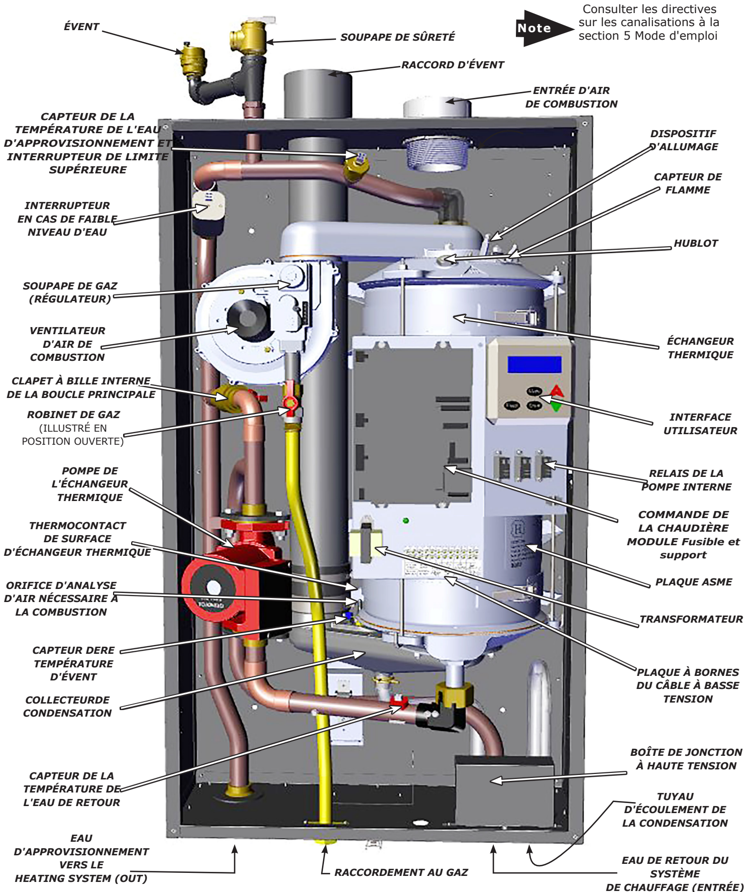
FIGURE 3-4 Composants de la chaudière 150-200 MBH (aperçu de l'avant de la chaudière)
