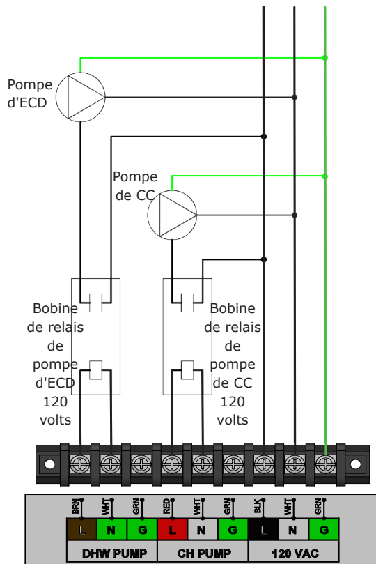
FIGURE 8-3 Relais d'isolation pour pompe du système de CC et pompe d'ECD
