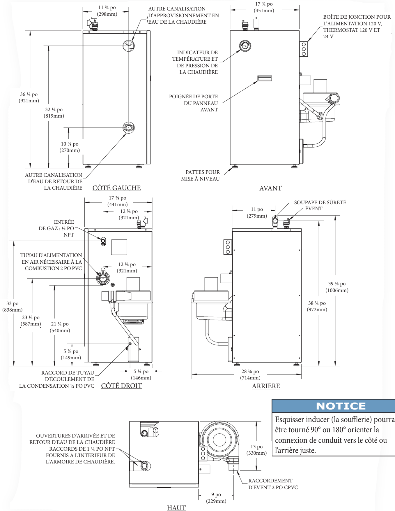
Figure 1 - Dimensions de la chaudière
