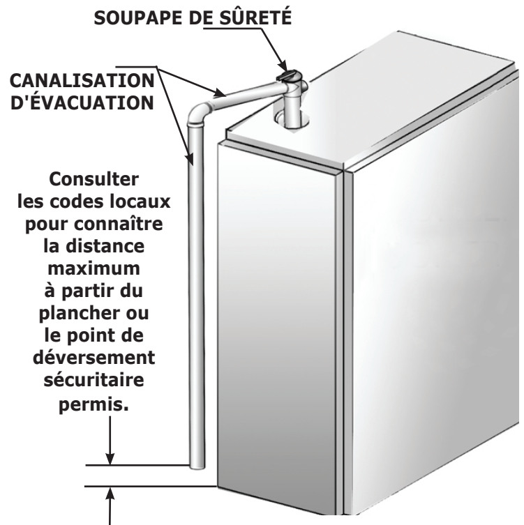
Figure 9 - Canalisation de la soupape de sûreté de la chaudière
