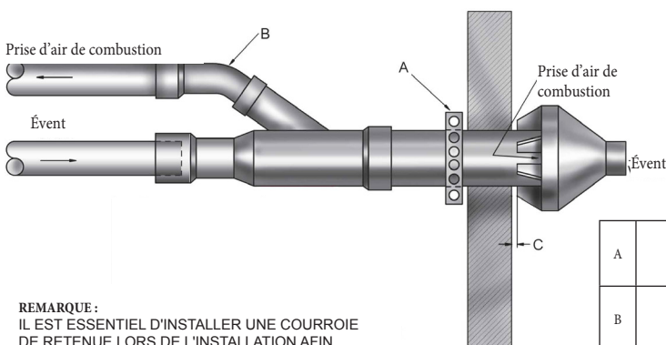
Figure 16 - Extrémités d'évent concentrique
