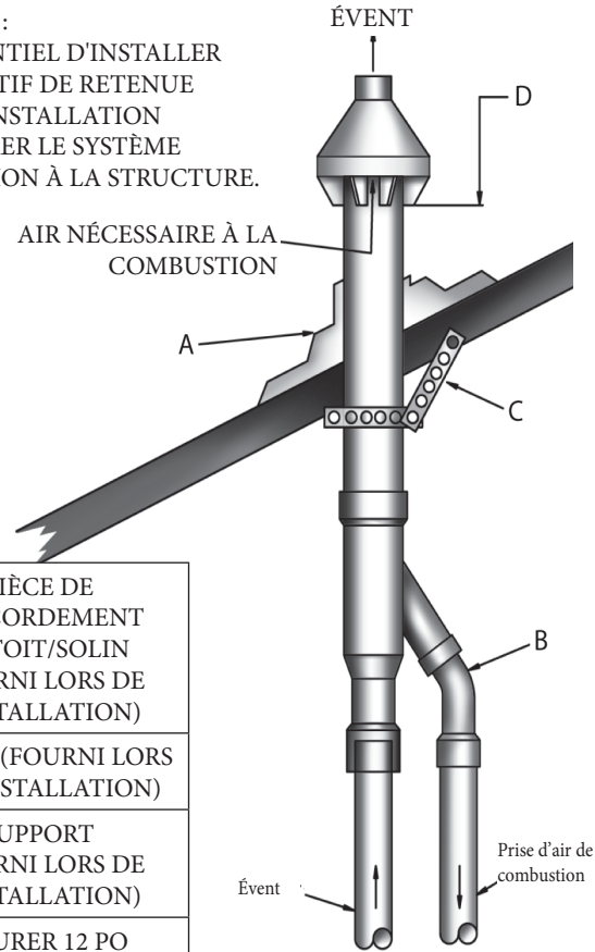
Figure 17 - Installation de l'évent concentrique sur le toit
