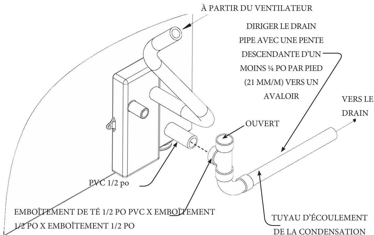
Figure 12 - Raccordements du vase d'expansion fermés conventionnels
