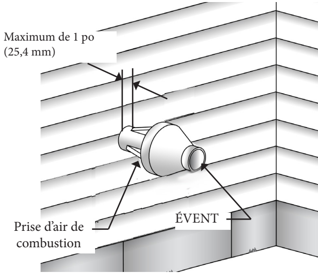
Figure 18 - Extrémités d'évent concentrique
