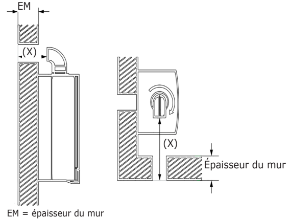
FIGURE 6-5 – Événement coaxial pour mur latéral
