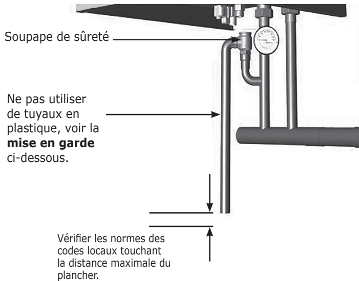
FIGURE 5-2 – Canalisation de sortie de la soupape de sûreté
