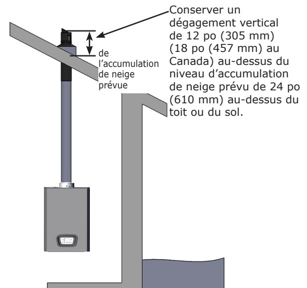
FIGURE 6-6 – Événement coaxial pour installation sur le toit
