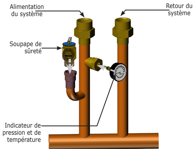
FIGURE 5-1 – Soupape de sûreté
