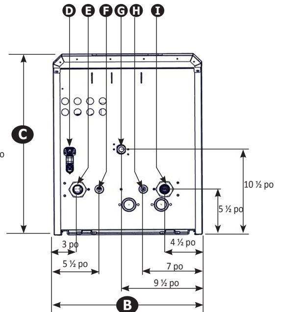
205 COMBI Vue de dessous Dimensions
