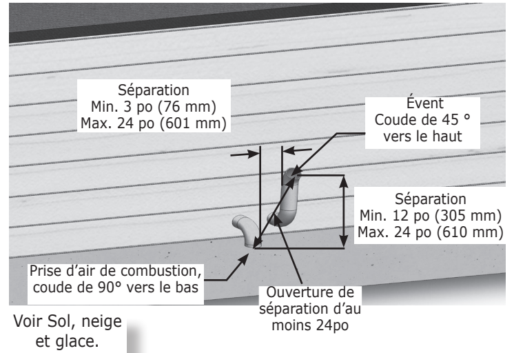
FIGURE 6-15 – Événement latéral de tuyau double avec angle de 45°
