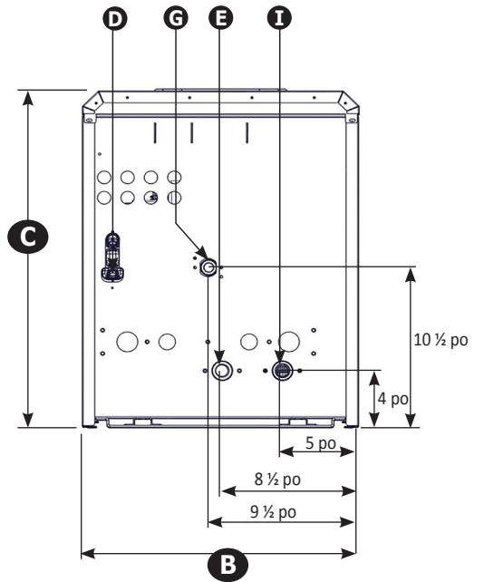
165 CHAUFFAGE SEULEMENT Vue de dessous Dimensions
