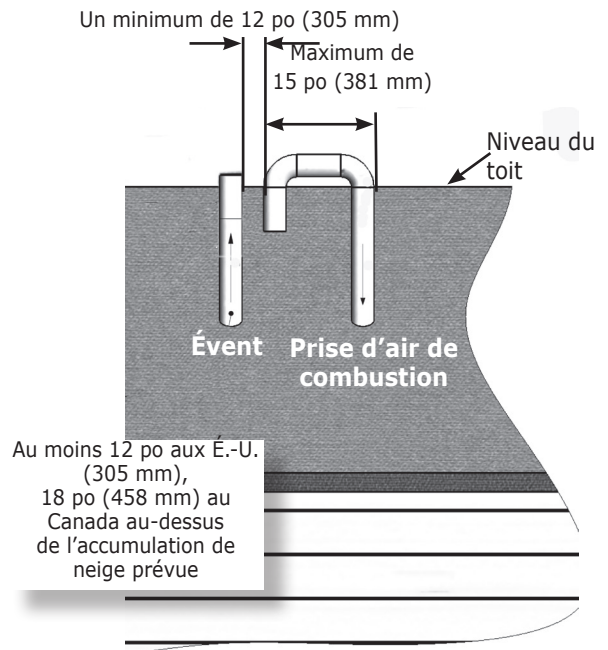
FIGURE 6-12 – Évent latéral de tuyau double (plusieurs appareils)
