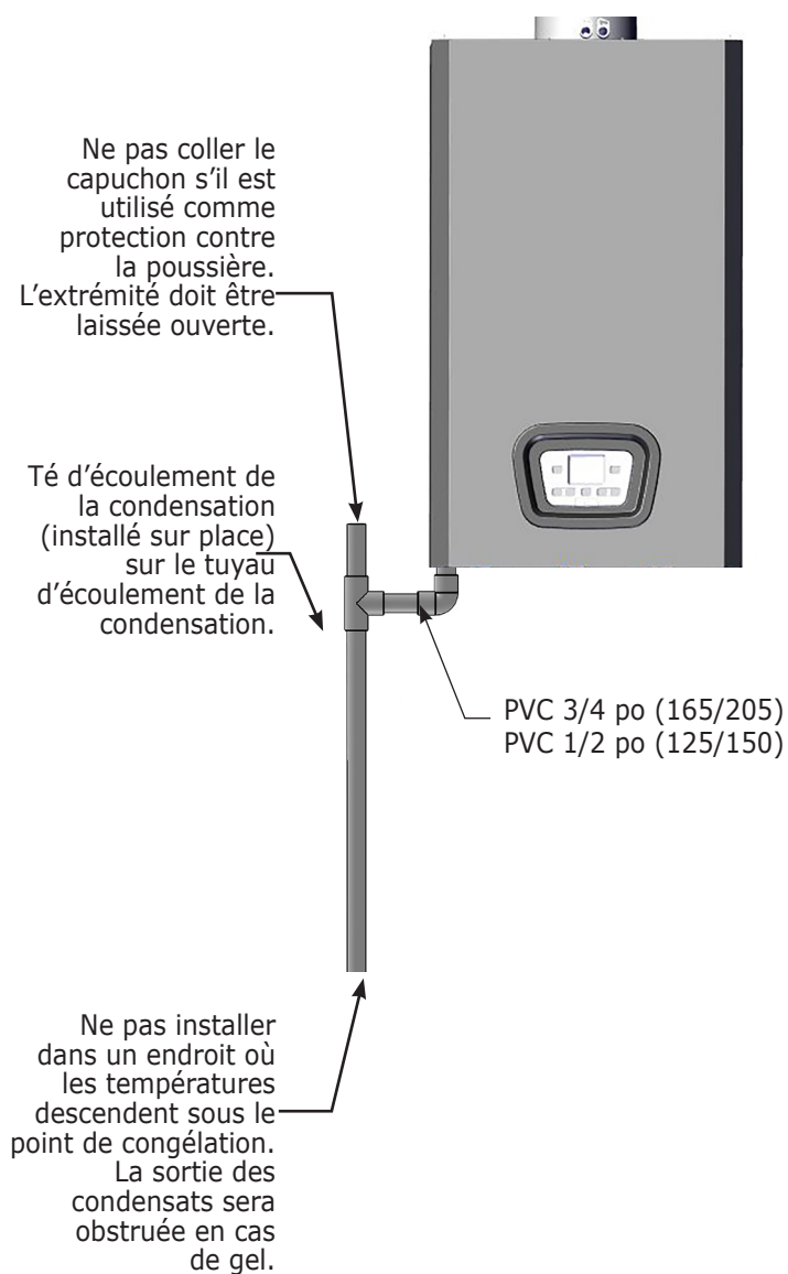
FIGURE 6-17 – Tuyau d’écoulement de la condensation
