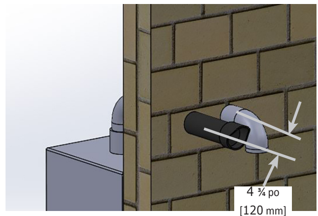
FIGURE 6-16 – Distance minimale d'un centre à l'autre entre l'adaptateur d'évacuation à paroi simple et la prise d'air
