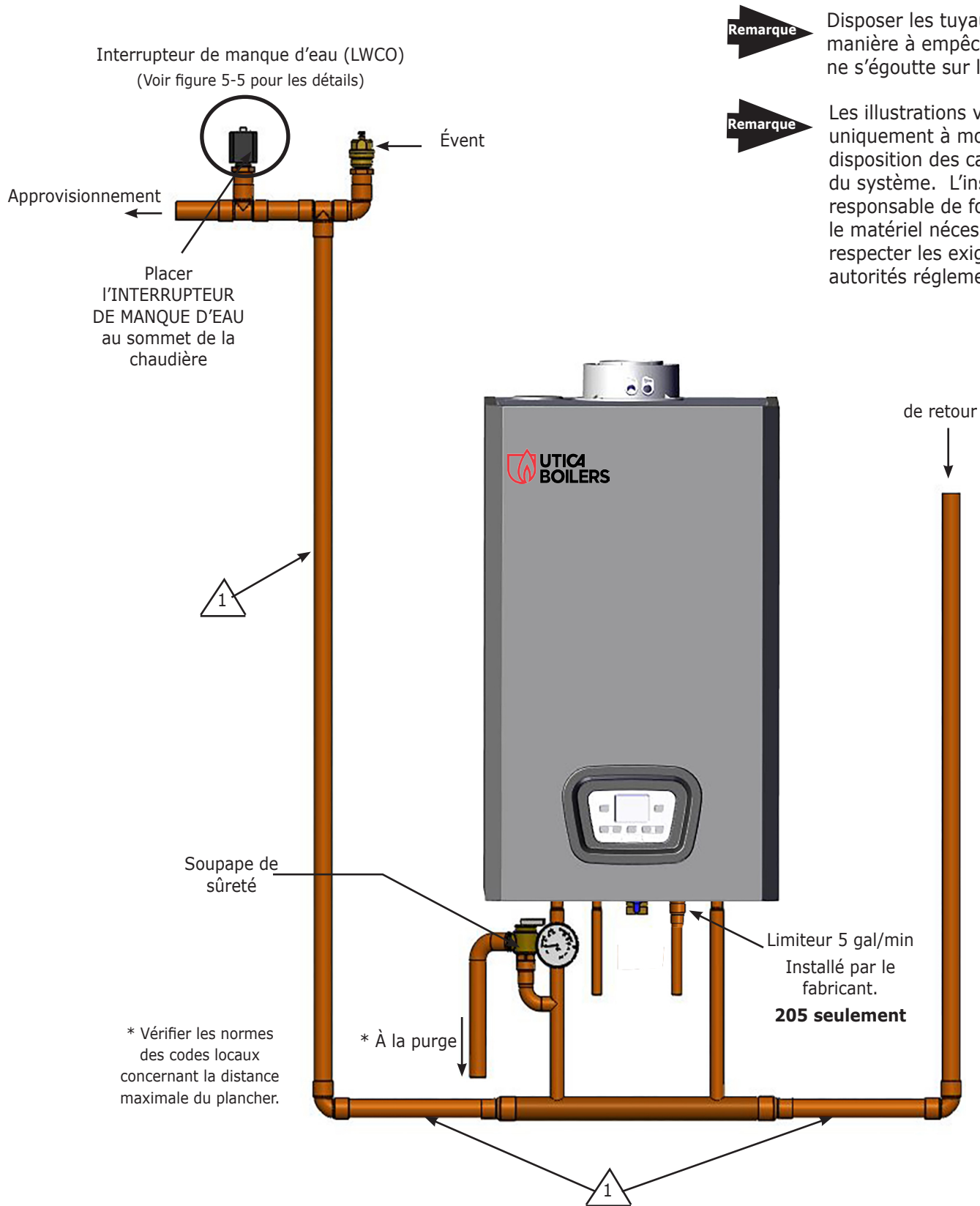
FIGURE 5-3 – Schéma des canalisations – Emplacement de l'interrupteur de manque d'eau
