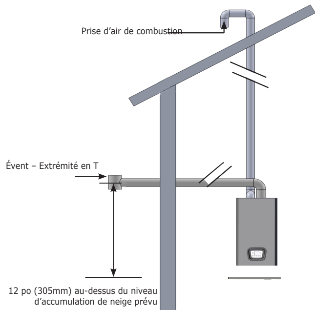
FIGURE 6-9 – Tuyau double d’évacuation sur le mur latéral, prise d’air nécessaire à la combustion sur le toit
