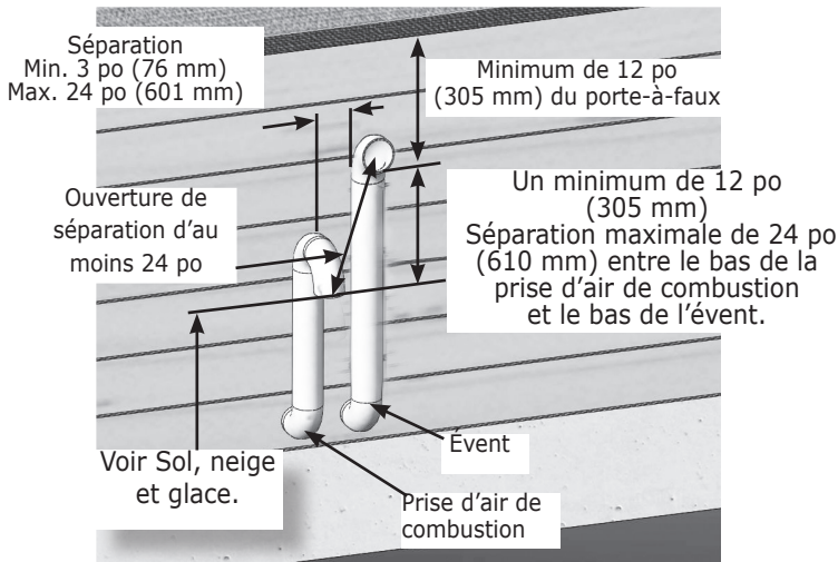
FIGURE 6-14 – Événement latéral de tuyau double
