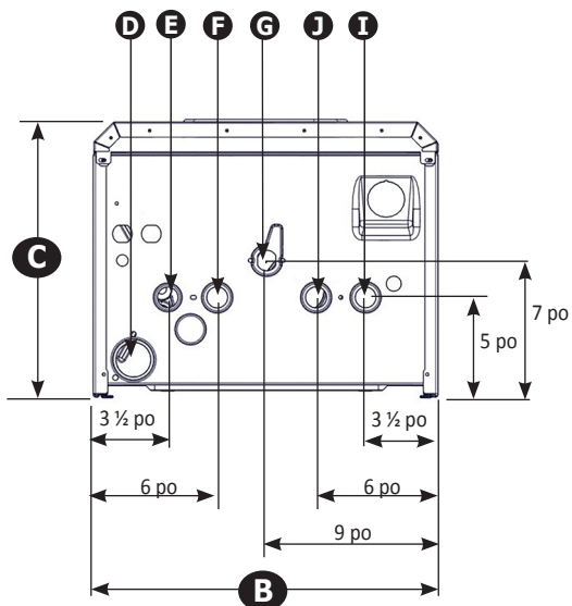
150 COMBI Vue de dessous Dimensions
