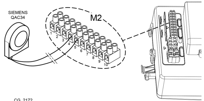
FIGURE 8-5 Raccordements au capteur extérieur
