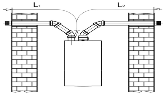
FIGURE 6-8 – Tuyau double sur le toit, prise d’air nécessaire à la combustion sur le mur latéral
