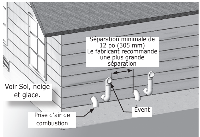
FIGURE 6-13 – Tuyau double horizontal, évacuation et prise d'air
